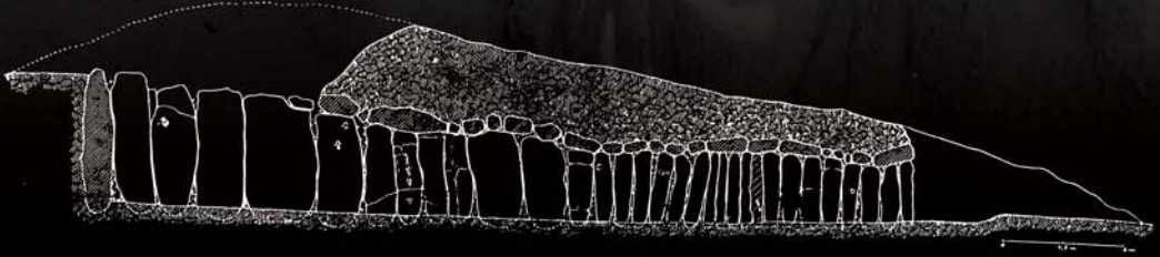
SECCIÓN LONGITUDINAL DERECHA.
